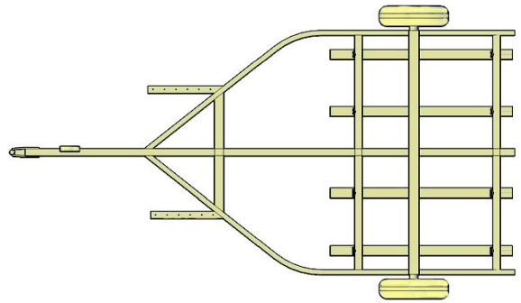
仰视图
