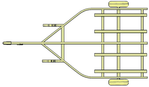
俯视图
